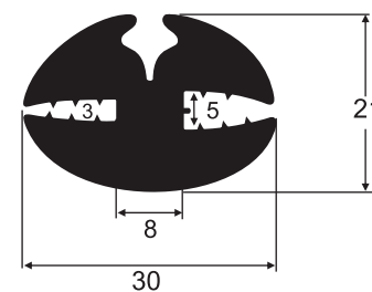
8017 SBR 60 Sh A Cunha 3119
