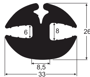
8079 EPDM 70 Sh A Cunha 3426
