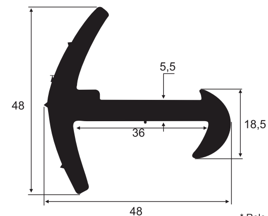
SBR 80 Sh A * SBR 85 Sh A * SBR 80 Sh A (Barra c/ 2,80 m) SBR 80 Sh A (Barra c/ 2,30 m) SBR 75 Sh A Vedação Porta Furgões
