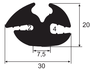
8079 EPDM 70 Sh A Cunha 3426
