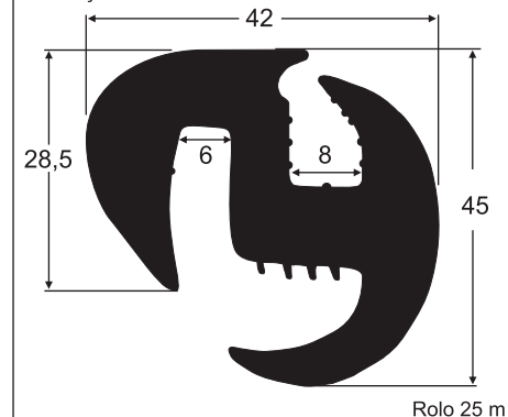
8024 EPDM 70 Sh A Guarnição Pára-brisa San Marino
