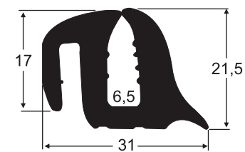
8027 EPDM 60 Sh A Guarnição Vidro Colheidadeira
