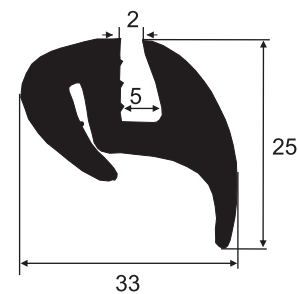
8026 EPDM 60 Sh A Vidro Porta San Marino
