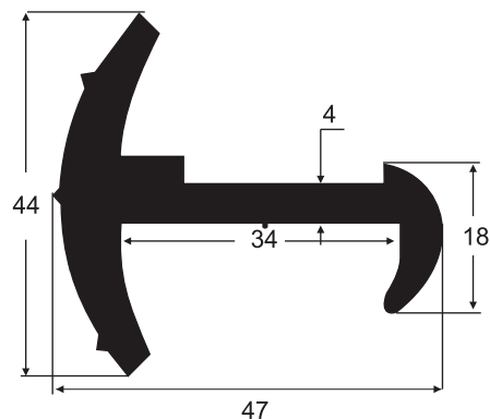
3223 SBR 85 Sh A Vedação Porta Furgões
