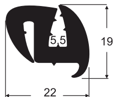
8019 SBR 60 Sh A Vigia do Mercedes Benz
