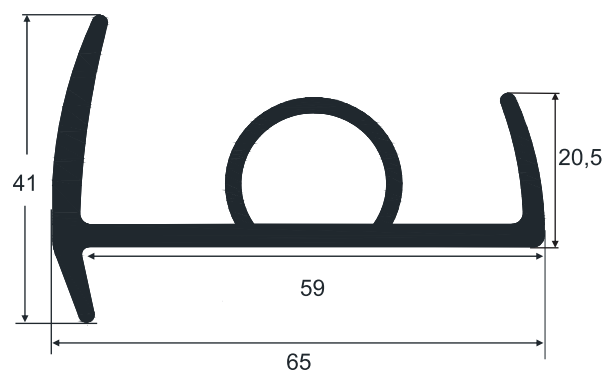
3592 EPDM 75 Sh A Vedação portas furgão HC
