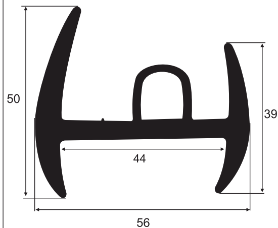
3306 EPDM 70 Sh A Vedação Caixa Rancho
