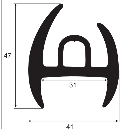
3306 EPDM 70 Sh A Vedação Caixa Rancho
