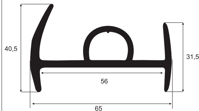
3592 EPDM 75 Sh A Vedação portas furgão HC
