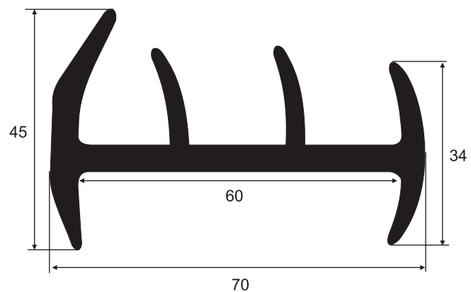
3536 EPDM 75 Sh A Vedação Porta Frigorífico
