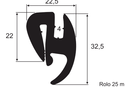
8024 EPDM 70 Sh A Guarnição Pára-brisa San Marino
