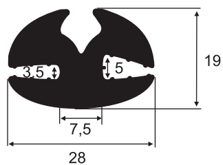
8060 SBR 60 Sh A Cunha 3101
