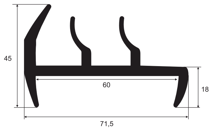
3538 EPDM 75 Sh A Vedação Porta Frigorífico
