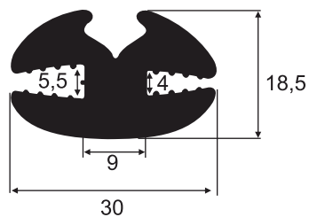
8016 SBR 60 Sh A Cunha 3101
