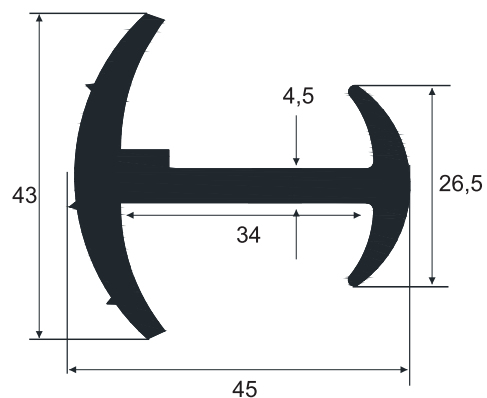
3038 SBR 80 Sh A Vedação Porta Furgões
