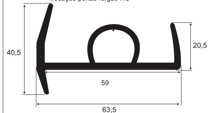
3310 EPDM 75 Sh A 7339 1.900mm. 7340 2.300mm. 7341 2.500mm. 7406 2.100mm. Vedação portas furgão HC
