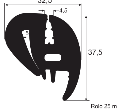
8021 SBR 60 Sh A Parabrisa MB - HPN - FPN
