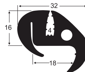
8026 EPDM 60 Sh A Vidro Porta San Marino
