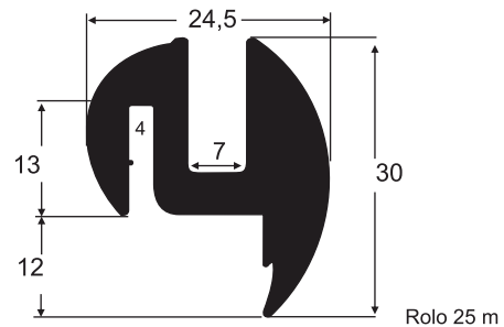
8021 SBR 60 Sh A Parabrisa MB - HPN - FPN
