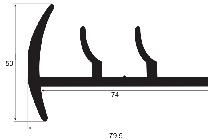
3413 EPDM 75 Sh A - Vedação Porta Frigorífico 3770 SBR 75 Sh A - Vedação Porta Frigorífico
