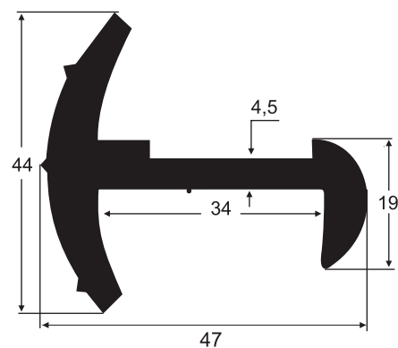
3223 SBR 85 Sh A Vedação Porta Furgões
